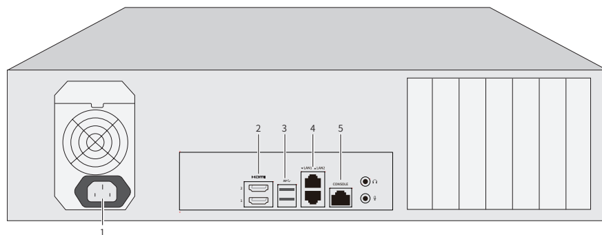
图1-3 TL-NVS7162-256后面板示意图
