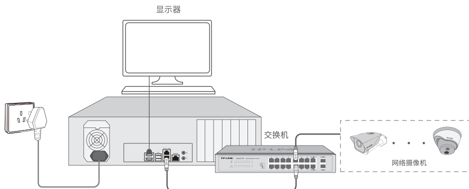
图3-6 单机状态NVS连接示意图
