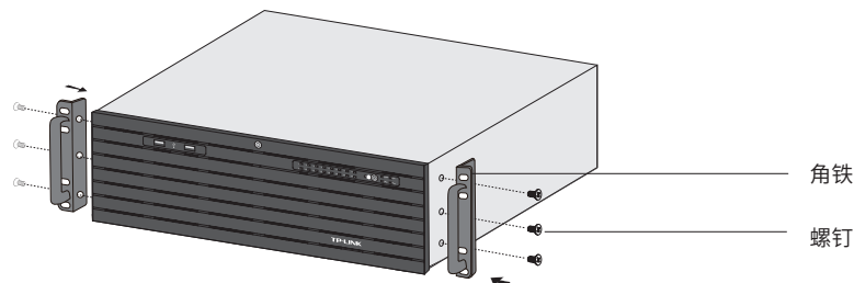
图2-1 角铁安装示意图
