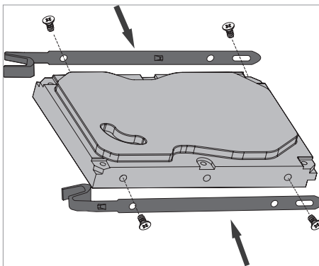
图3-2 安装硬盘支架
